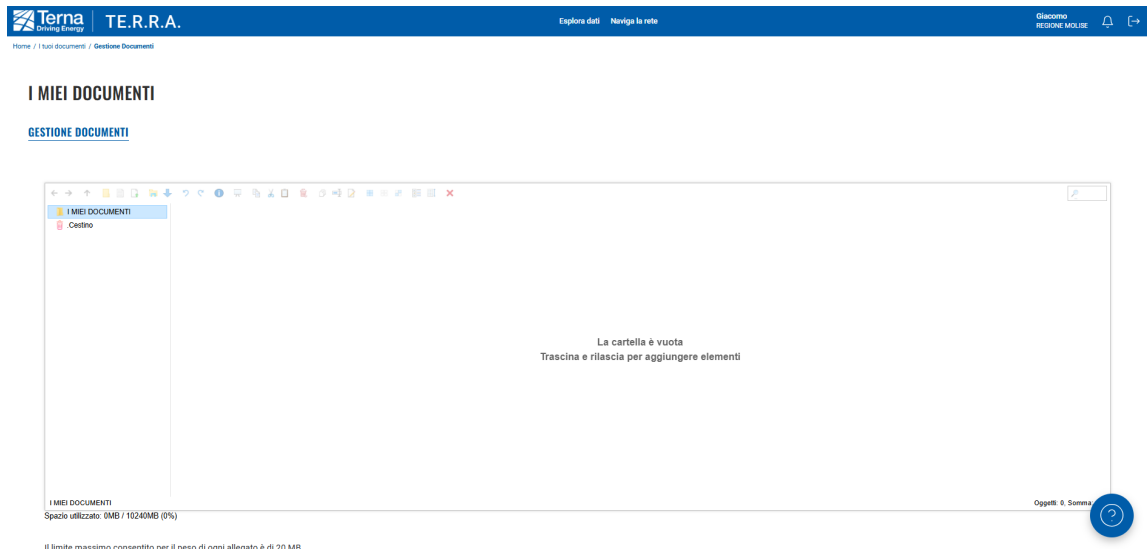
Figura 145: Gestione documenti
